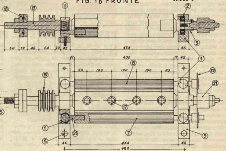
FIG. 1d PIANTA
