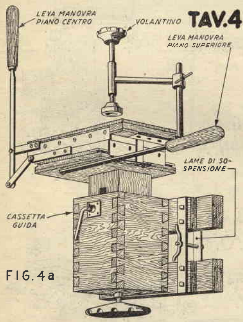
SCHIZZO PROSPETTICO CAVATRICE (AFFILATRICE)
