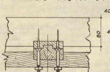
FIG. 2e PARTICOLARE GUIDE PIANO INFER. SEZ. ORIZZ. B
