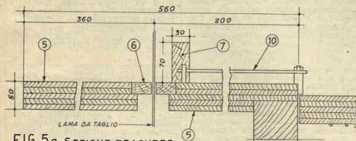
FIG.5e SEZIONE TRASVERS. PARTICOLARE
