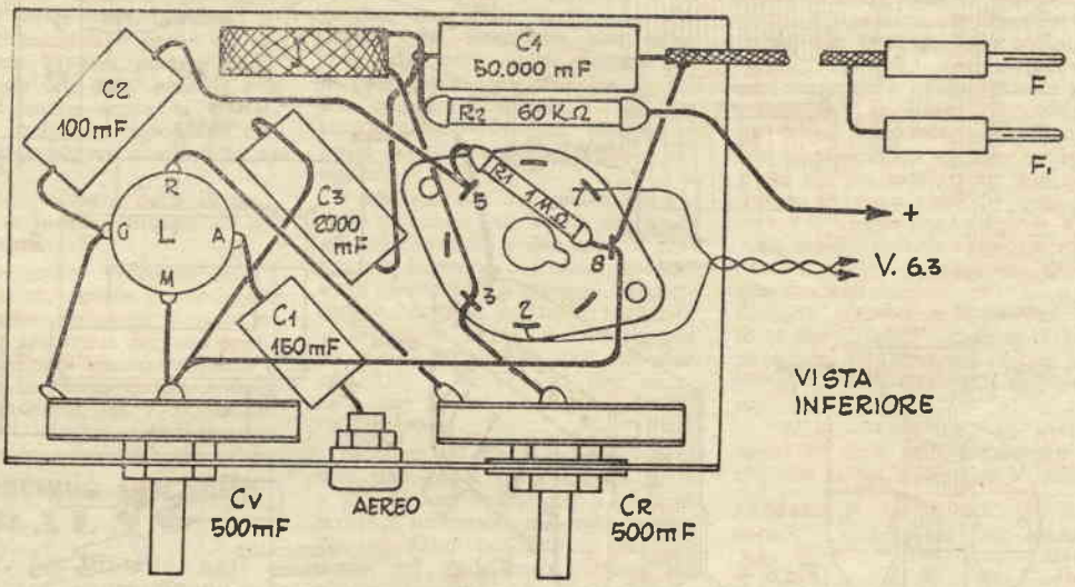
Fig. 4 SCHEMA COSTRUTTIVO
