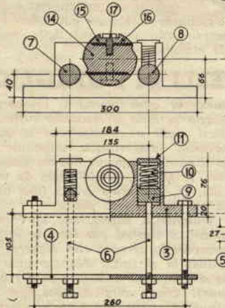
FIG. 1c FIANCO SEZIONATO
