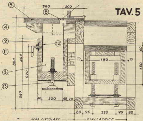
FIG.5d. SEZIONE TRASVERSALE
