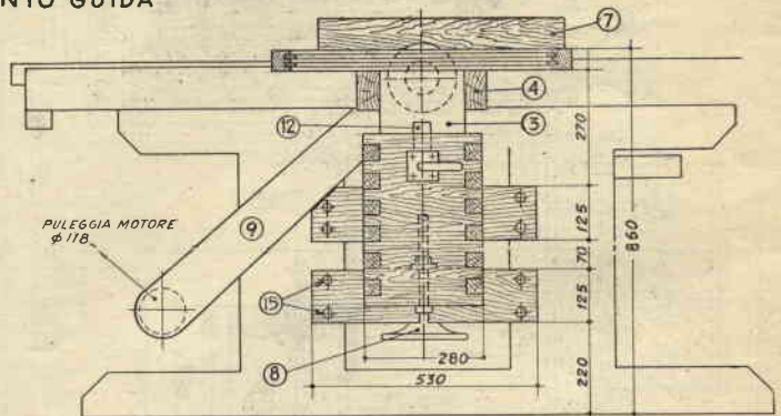
FIG. 5b FRONTE
